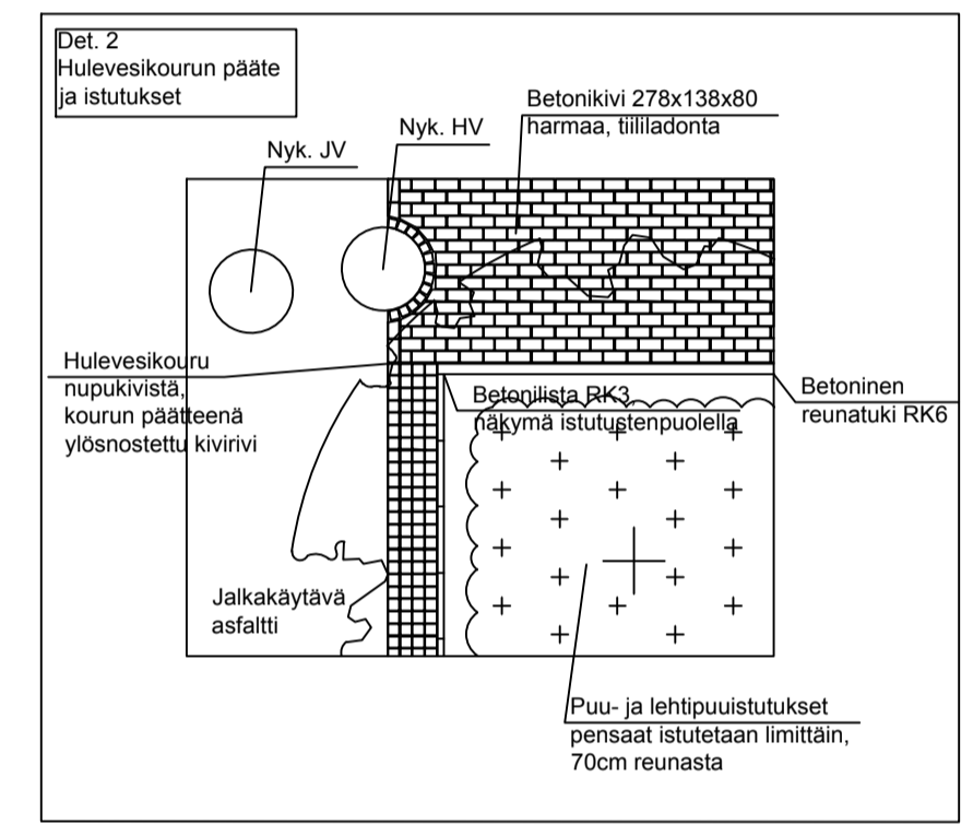
Detalji 2 Hulevesikourun pääte ja istutukset 1:100
