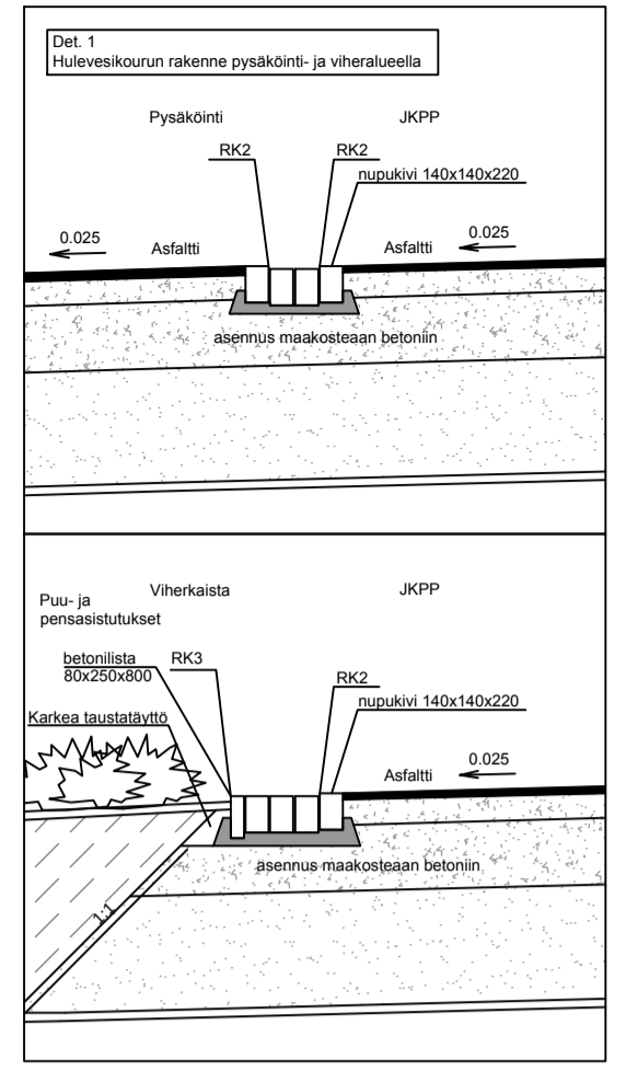
Detalji 1 Hulevesikourun rakenne pysäköinti- ja viheralueella 1:50
